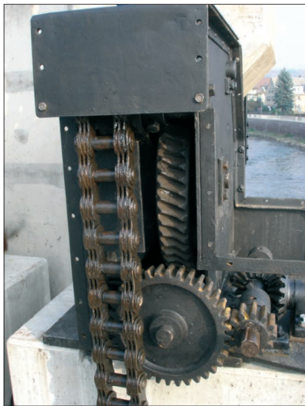
Einblick in die einfache und gut funktionierende Wehrtechnik – Blick in den Getriebekasten. Bild: Archiv Christian Rößler
